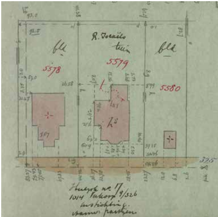
Kadaster, Veldwerk_ODN00_D_344_1. Op deze veldwerktekening uit 1927 staan de maten van de kavel en van het huis van Rafel Israëls (D5579) vermeld.
